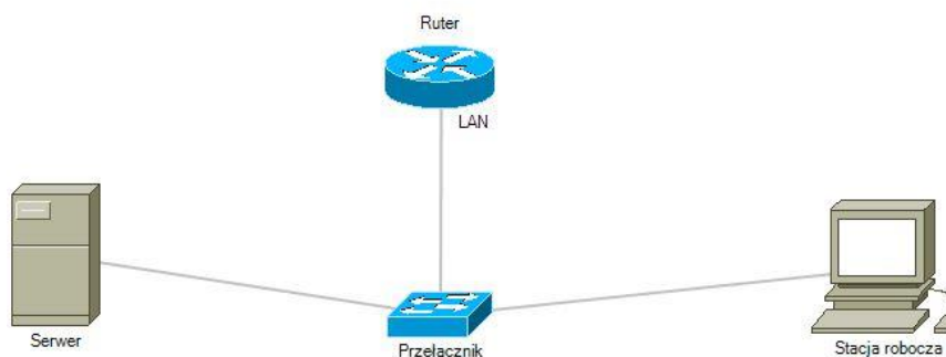
Schemat połączenia urządzeń
